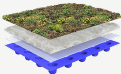
Lichtgewicht groendak | 40-45 kg/m 2
